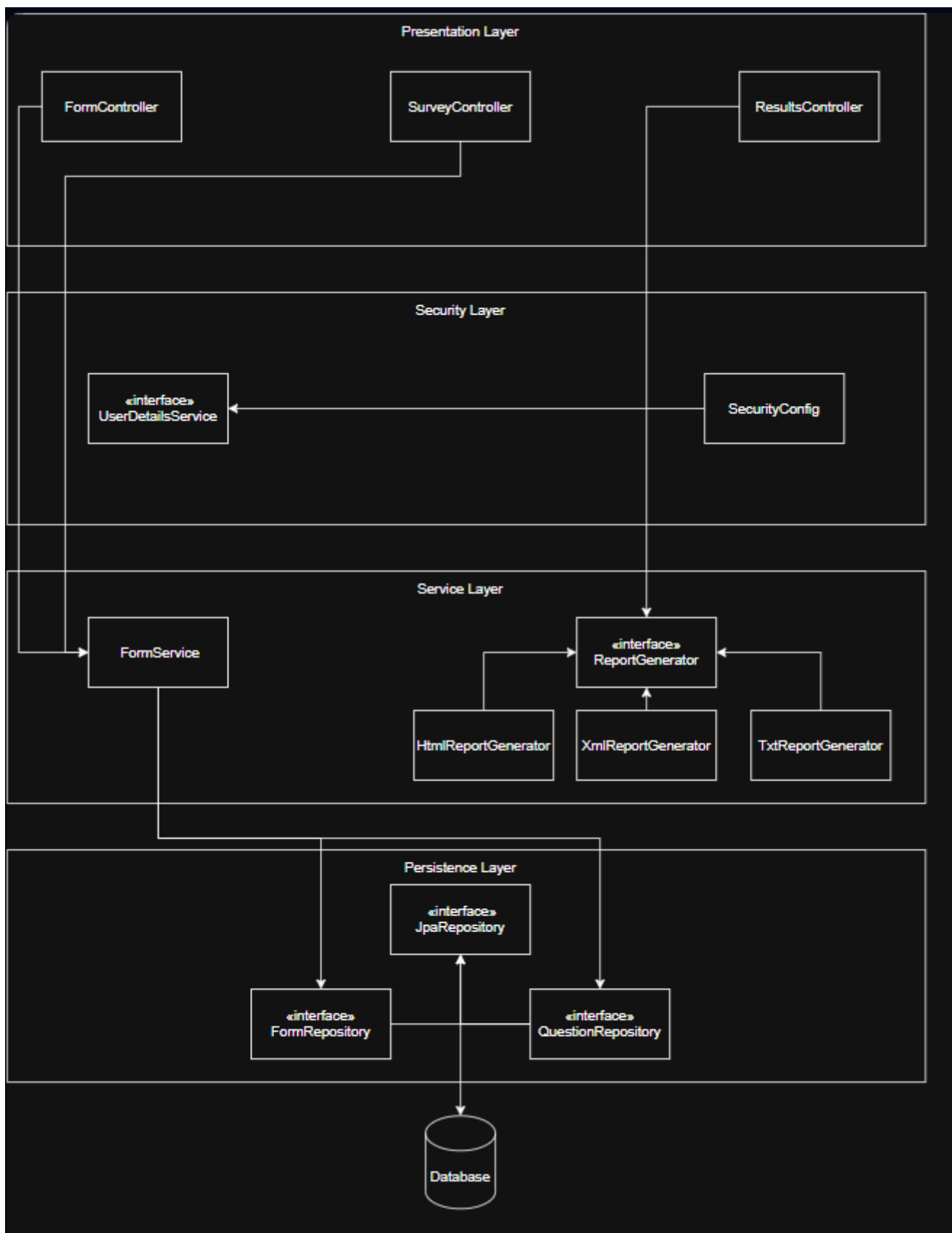
Рисунок 5 - Схема взаимодействия программных Java интерфейсов и слоев
