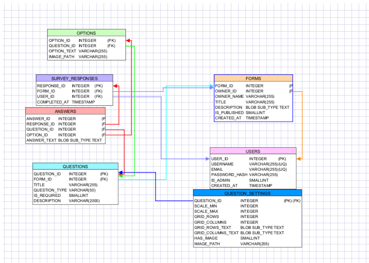
Рисунок 6 – ER-диаграмма
